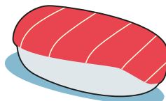
NIGIRI
