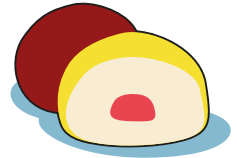
MOCHI
