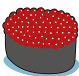
GUNKAN
