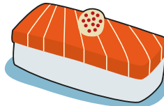
BATTERA
